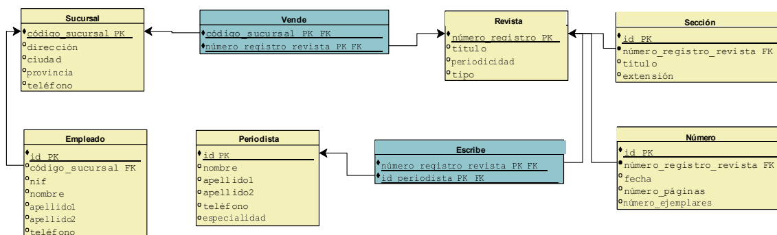
ILUSTRACIÓN 4. DIAGRAMA RELACIONAL
