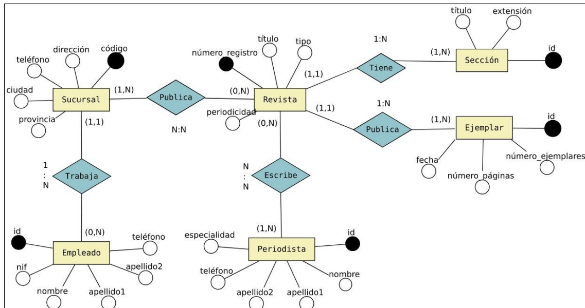
ILUSTRACIÓN 3. DIAGRAMA E/R
